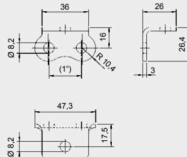
For chains M 1610 A und M 1611 SL: Design 202.13
