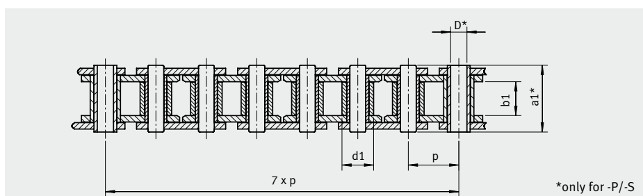
iwis POChain-P
